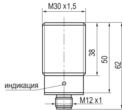
Габаритный чертеж
